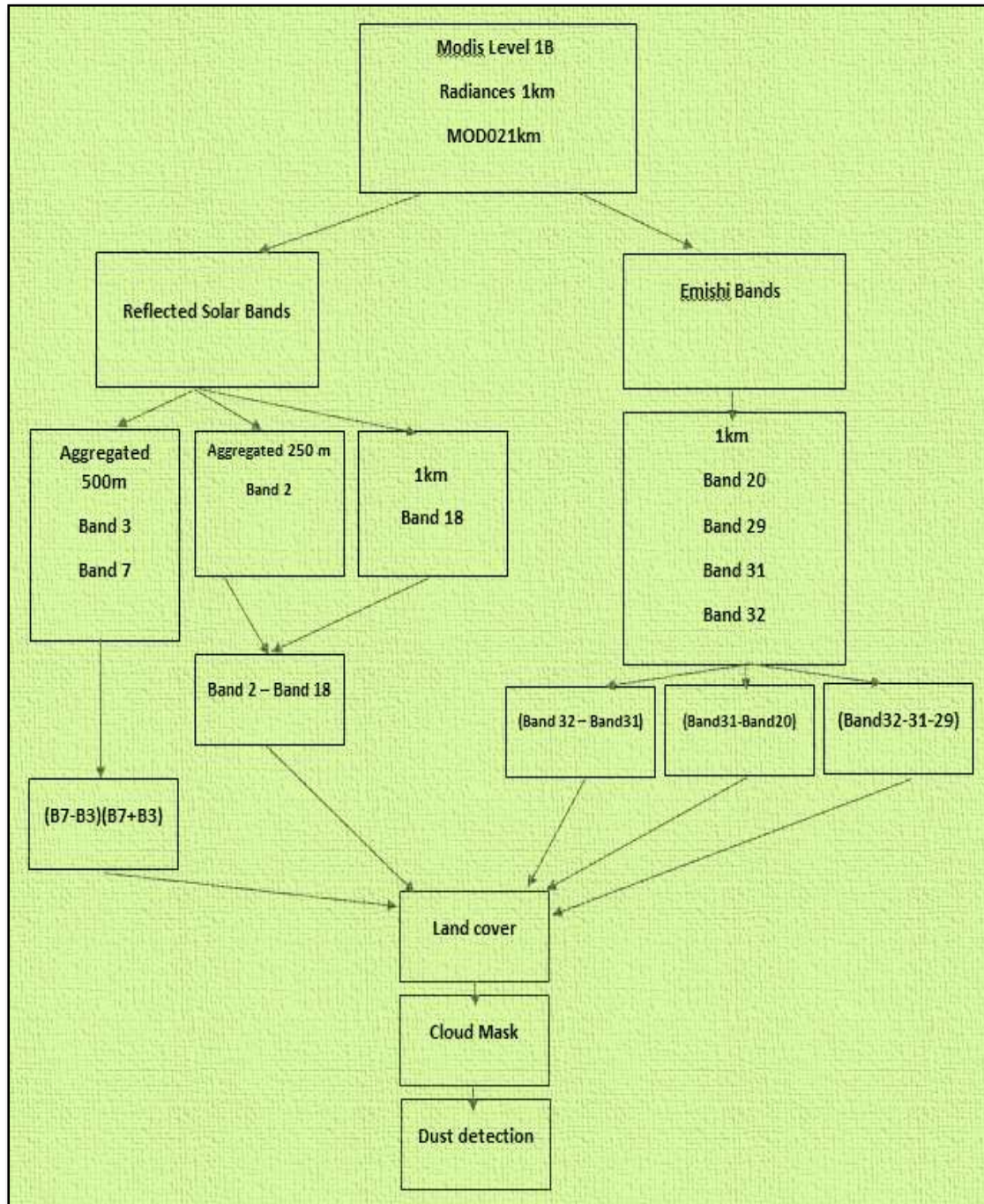
الشكل (٢) طرائق اعداد نموذج استخلاص مؤشر العواصف الغبارية من (MODIS)
