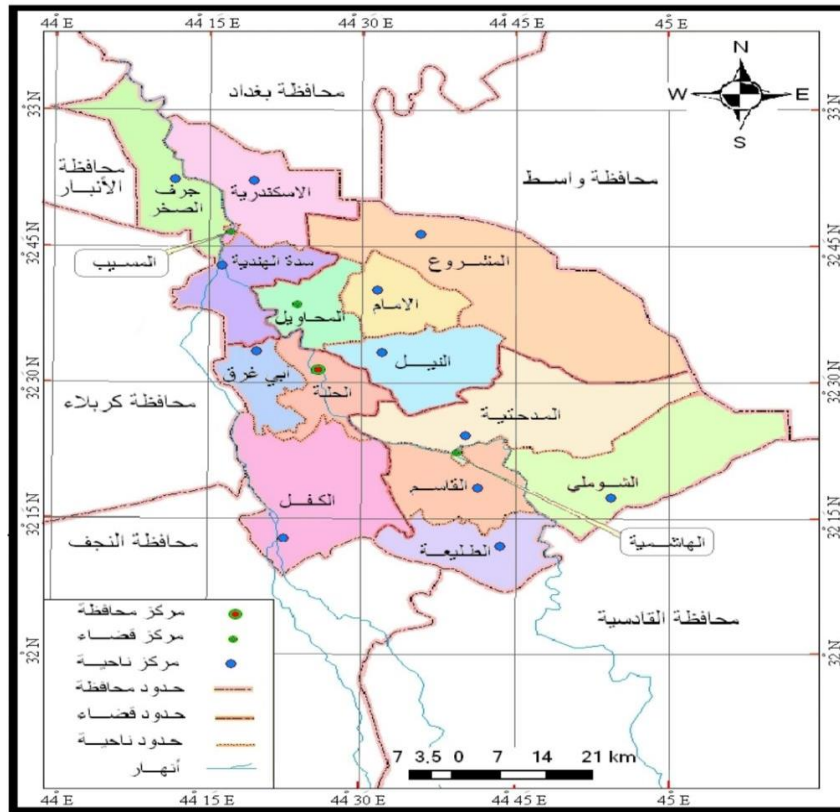
خارطة (٢) الوحدات الادارية لمحافظة بابل
