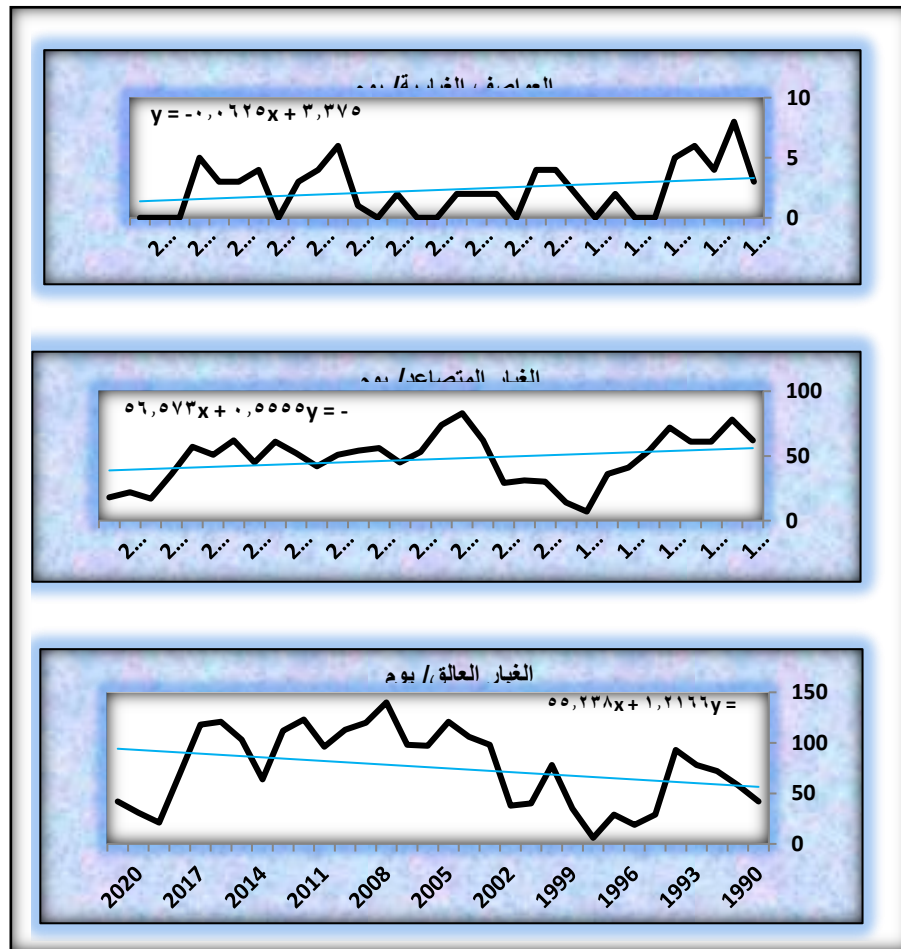
شكل (٨) الاتجاه العام للمجموع السنوي للظواهر الغبارية لمحطة الحلة
