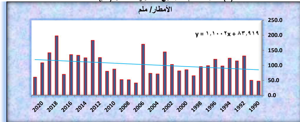
شكل (٧) الاتجاه العام للمجموع السنوي للأمطار (ملم) لمحطة الحلة
