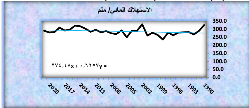
شكل (١٤) الاتجاه العام السنوي للاستهلاك المائي لمحصول القربيط لمحطة الحلة
