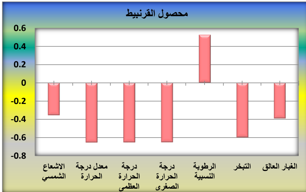
شكل (١٧) العناصر والظواهر المؤثرة على كمية إنتاج محصول القرنبيط لمحطة الحلة
