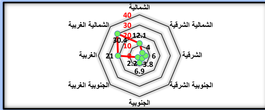
شكل (٤) اتجاه الرياح في محطة الحلة للمدة (١٩٩٠ - ٢٠٢٢) م
