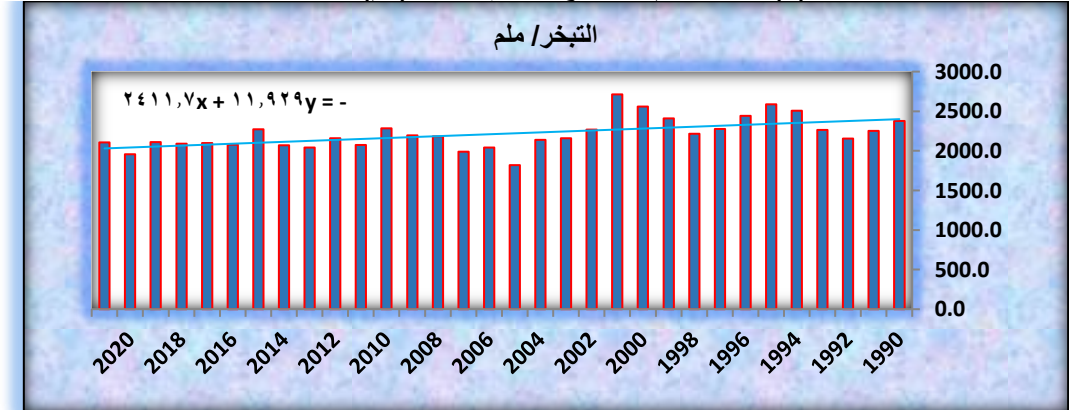
شكل (٦) الاتجاه العام للمجموع السنوي للتبخر (ملم) لمحطة الحلة
