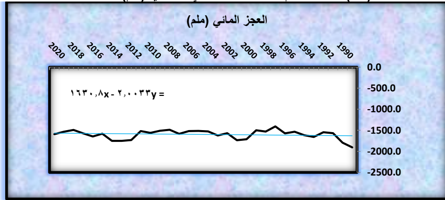
شكل (١١) الاتجاه العام لكمية العجز المائي السنوي (ملم) لمحطة الحلة
