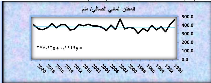
شكل (١٦) الاتجاه العام السنوي للمقنن المائي الصافي لمحصول القربيط لمحطة الحلة
