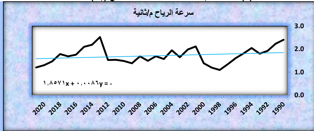
شكل (٣) الاتجاه العام للمعدلات السنوية لسرعة الرياح (م/ثا) لمحطة الحلة
