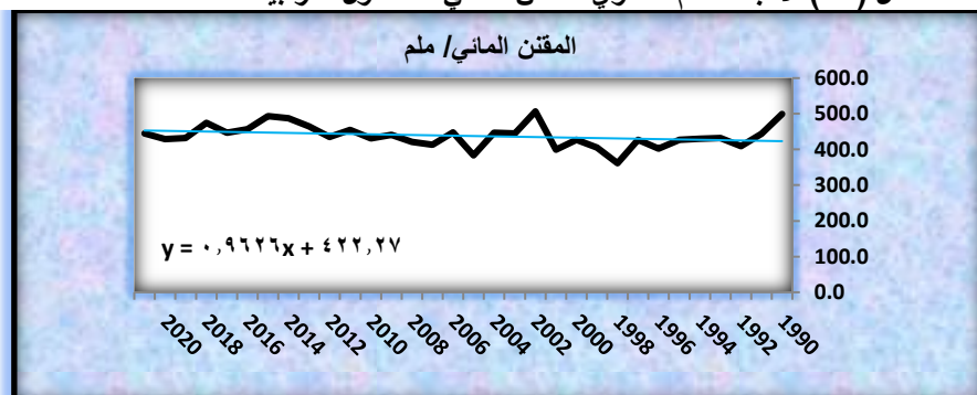
شكل (١٥) الاتجاه العام السنوي للمقنن المائي لمحصول القربيط لمحطة الحلة
