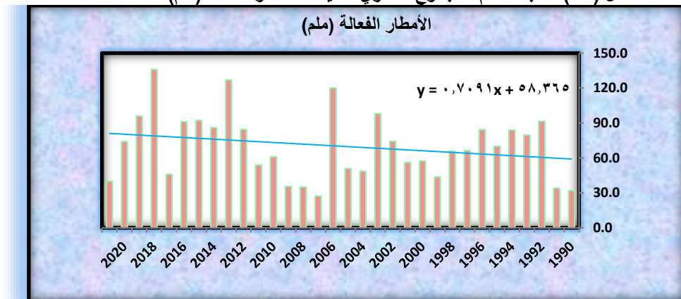
شكل (١٠) الاتجاه العام للمجموع السنوي لكميات الأمطار الفعالة (ملم) لمحطة الحلة
