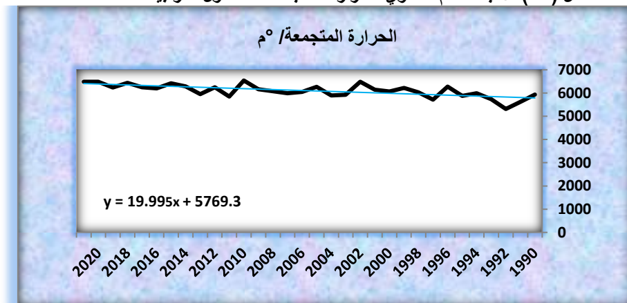
شكل (١٣) الاتجاه العام السنوي للحرارة المتجمعة لمحصول القربيط لمحطة الحلة
