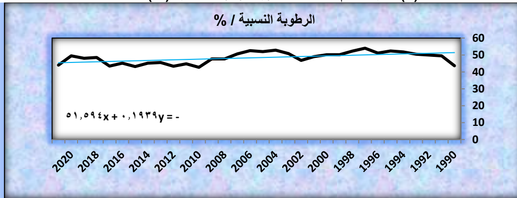
شكل (٥) الاتجاه العام للمعدلات السنوية للرطوبة النسبية (%) لمحطة الحلة
