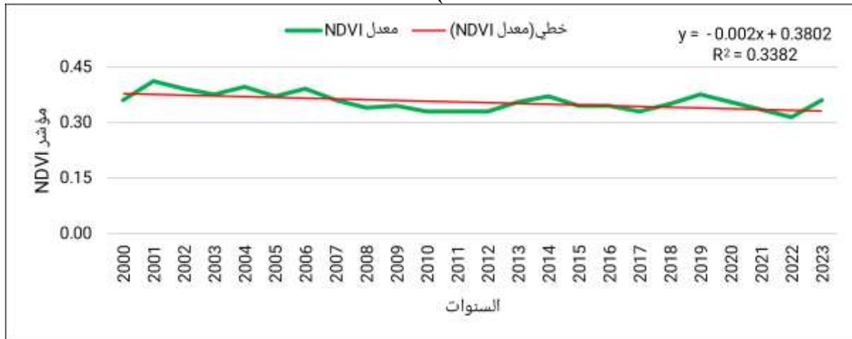
الشكل (2) قيمة الانحدار السنوي لمؤشر NDVI في المناطق البساتين للمدة من (٢٠٠٠ - ٢٠٢٣)
