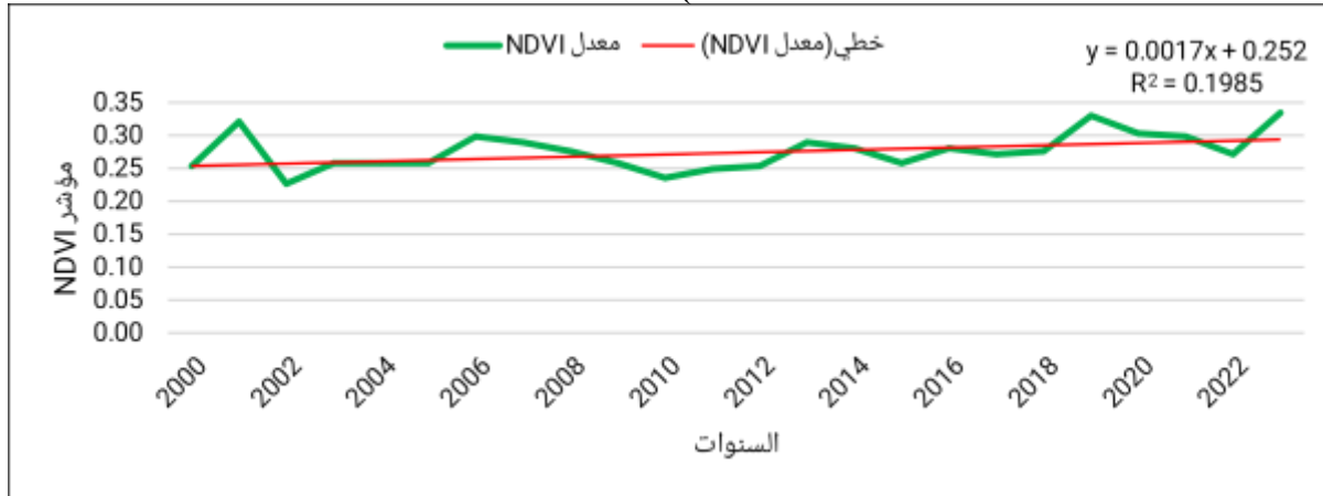
الشكل (١) قيمة الانحدار السنوي لمؤشر NDVI في المناطق الزراعية للمدة من (٢٠٠٠ - ٢٠٢٣)
