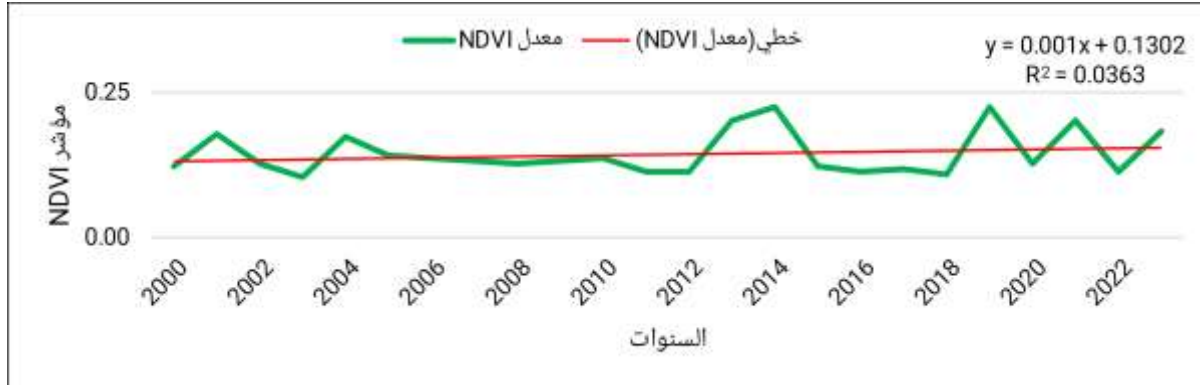
الشكل (٦) قيمة الانحدار السنوي لمؤشر NDVI في مناطق الفيضات للمدة من (٢٠٠٠ - ٢٠٢٣)
