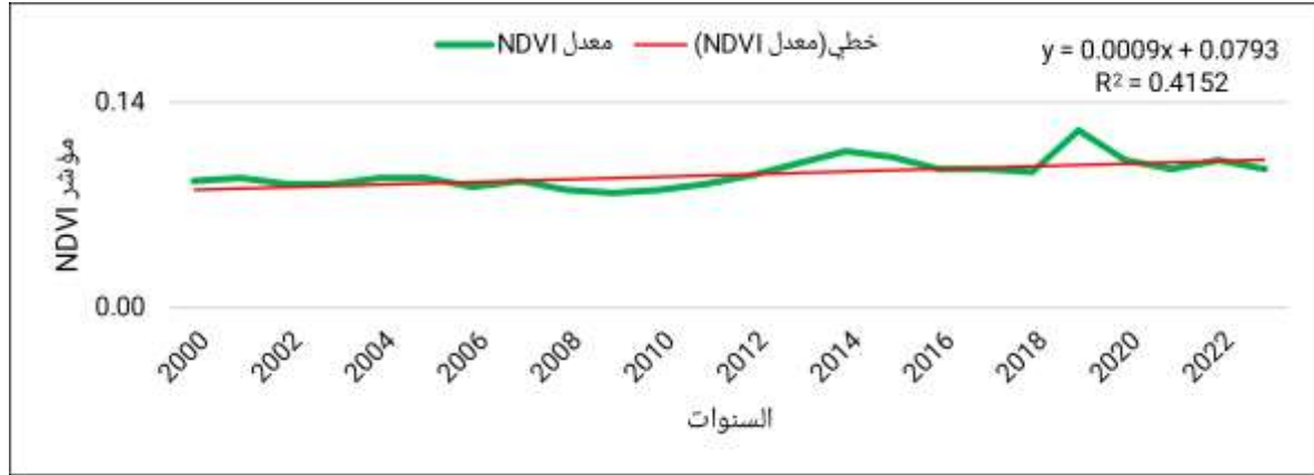
الشكل (٣) قيمة الانحدار السنوي لمؤشر NDVI في المنطقة الملحية للمدة من (٢٠٢٣ - ٢٠٠٠)
