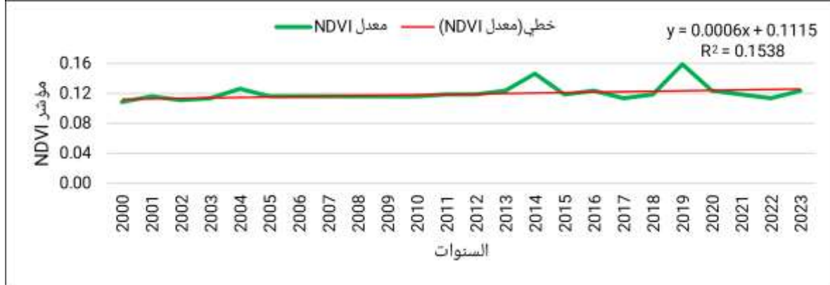
الشكل (٤) قيمة الانحدار السنوي لمؤشر NDVI في المنطقة الرعوية للمدة من (٢٠٠٠ - ٢٠٢٣)
