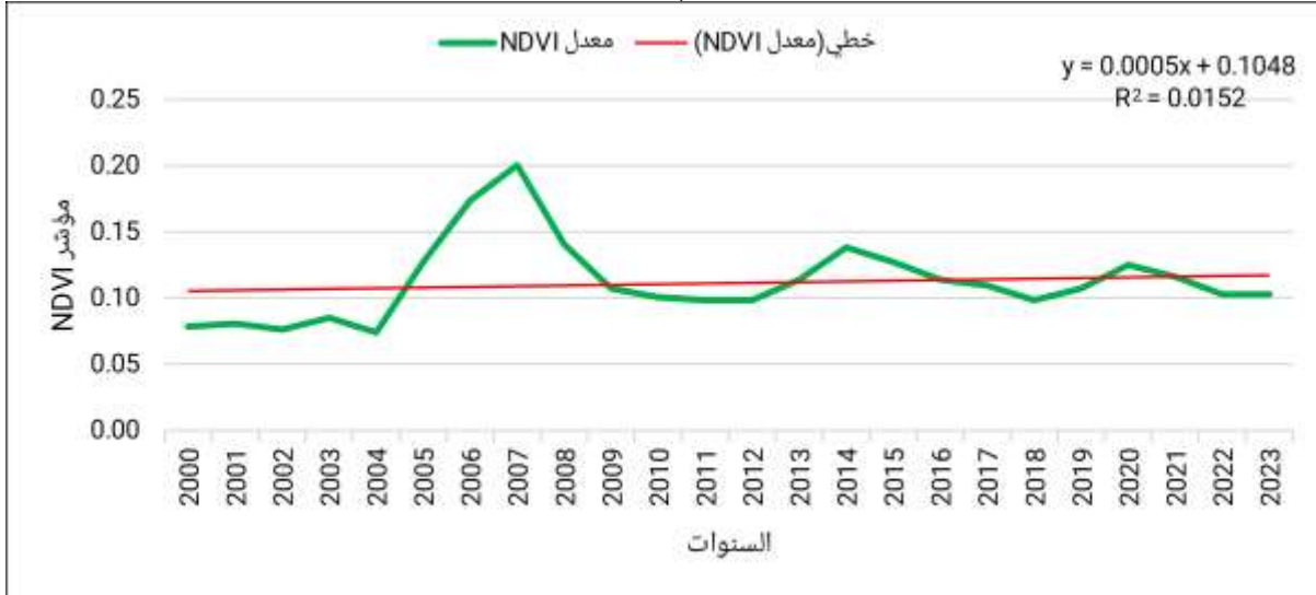
الشكل (٥) قيمة الانحدار السنوي لمؤشر NDVI في منطقة الاهوار للمدة من (٢٠٠٠ - ٢٠٢٣)
